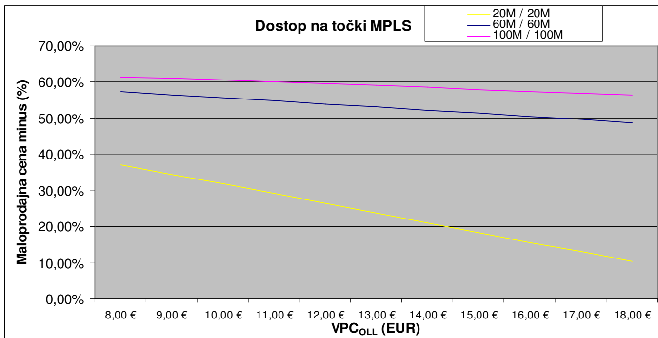
Slika 40: Maloprodajna cena minus (v %) na nivoju IP/MPLS za posamezne hitrosti
