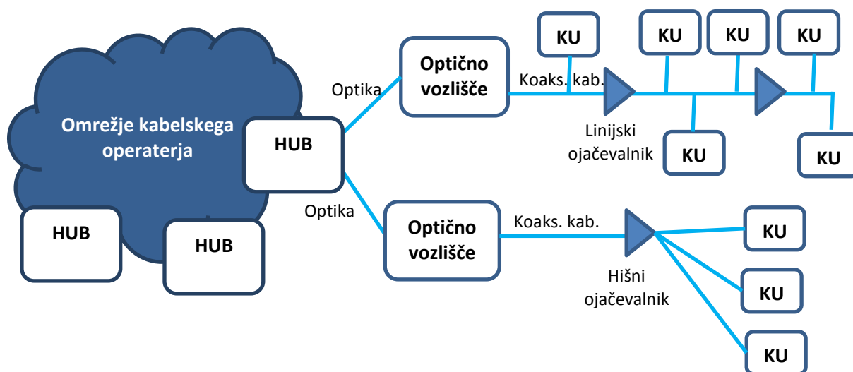
Shema kablanskega omrežja
