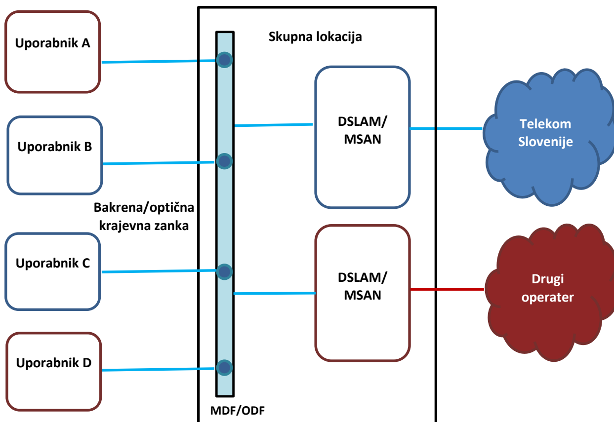
Slika 20: Fizična razvezava krajevne zanke
